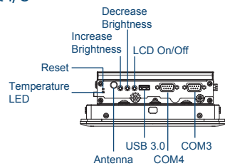
Left I/O
