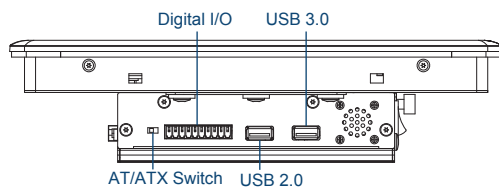
Left I/O
