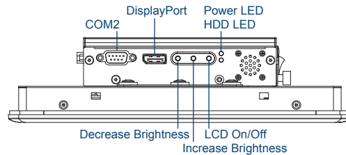
Right I/O
