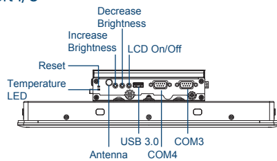
Left I/O
