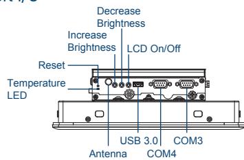
Left I/O
